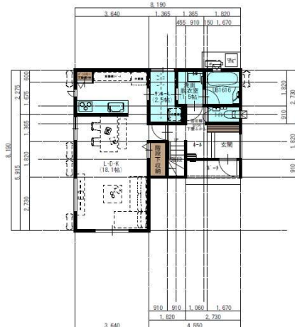
■ 1 階平面図 ■
